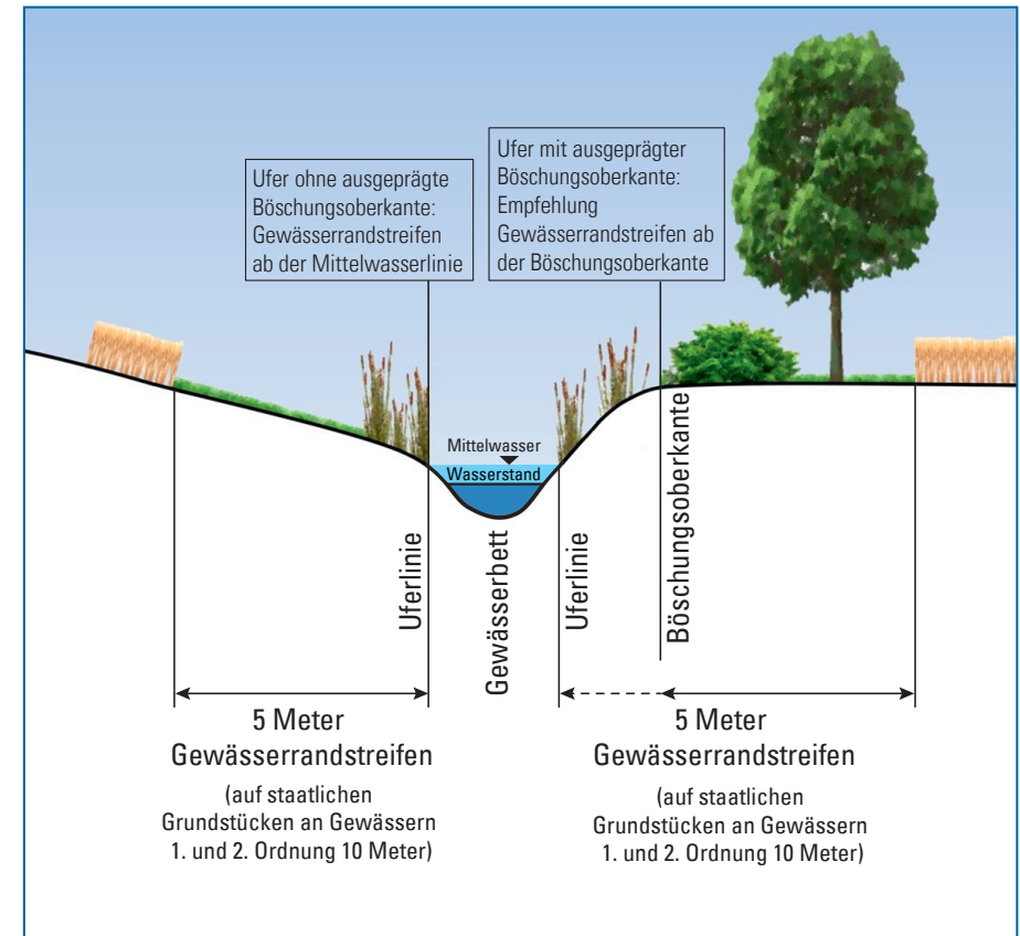
Beispielhafte Darstellung des Gewässerrandstreifens
